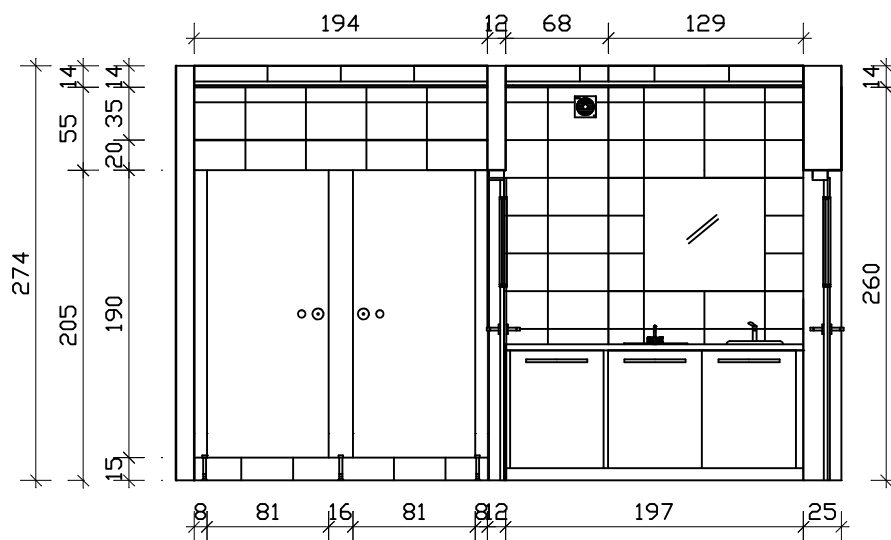
RYSUNEK NR 2 - PRZEKRÓJ A-A
