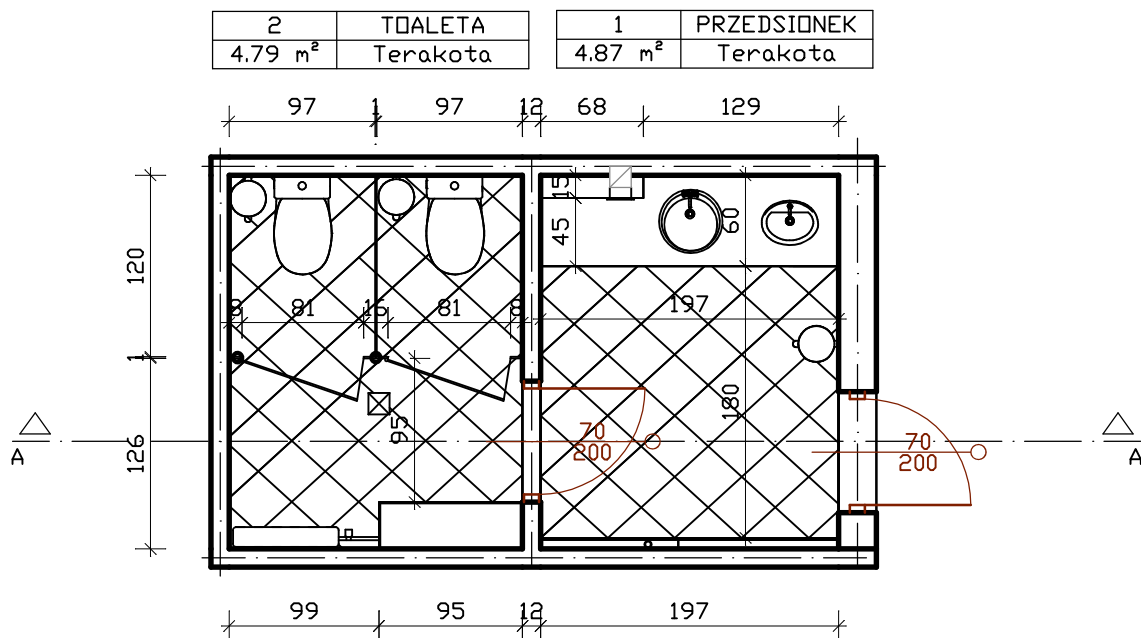
RYSUNEK NR 1 - RZUT TOALETY
